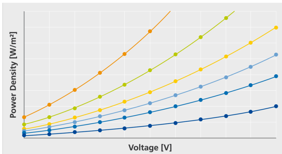
Densità di potenza e tensione di alimentazione
