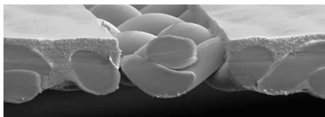
Contorno definido, superfície de impressão retangular, com SEFAR® PCF FC 180/460-27Y, 3 µm EOM
