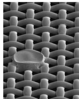
Adhérence du pochoir avec tissu polyester courant 120/305-34Y
