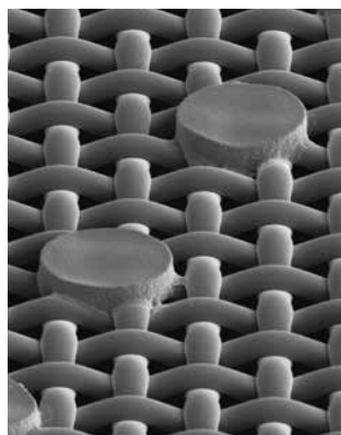
Adhérence du pochoir avec SEFAR® PET 1500 120/305-34Y
