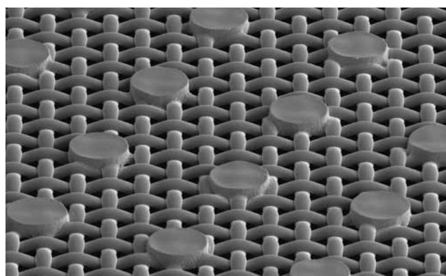
Surface de tissu optimisée en termes d'adhérence – SEFAR® GLASSLINE 77/195-55Y
