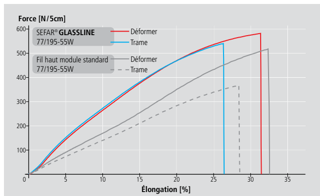
Force maximale d'allongement à la rupture SEFAR® GLASSLINE 77/195-55W
